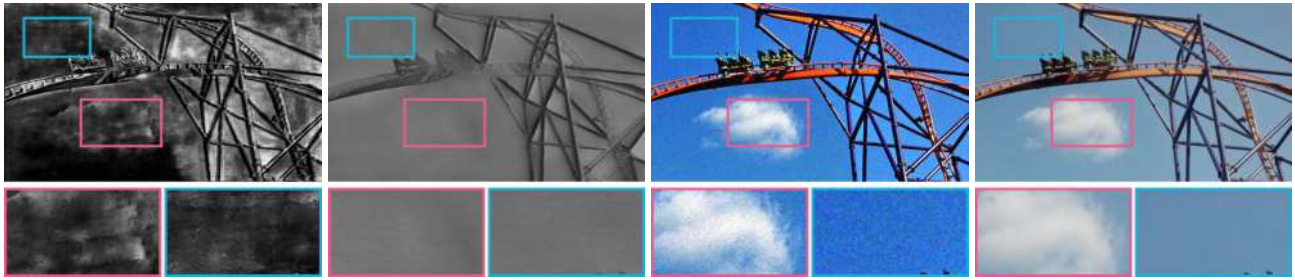
(d) DVS-Dark [21]
